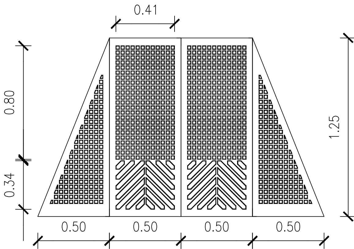
PLANTA
